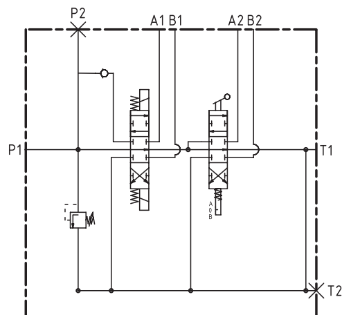
Versione V5 elettrica: priorità 1 sez. ed interruzione alimentazione delle sezioni a valle 12Vcc o 24Vcc (V5 (12V); V5 (24V))
